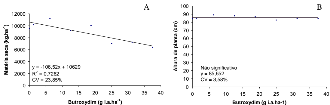
FIGURA 2: Efeito da deriva de butoxydim na produção de matéria seca e na altura de plantas de arroz, CAP-UFPel, Capão do Leão-RS, 200/01.
