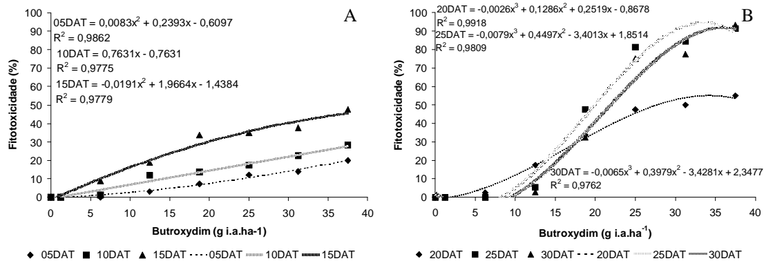
FIGURA 1: Fitotoxicidade observada em plantas de arroz submetidas a subdoses do herbicida butoxydim, CAP-UFPel, Capão do Leão-RS, 2000/01.
