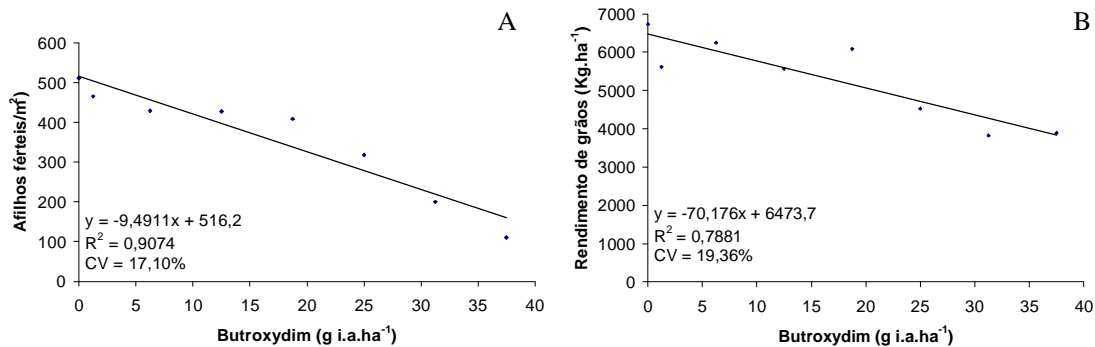
FIGURA 3: Efeito da deriva de butroxydim no número de afilhos férteis, no número de grãos por panícula, no peso de mil grãos e no rendimento de grãos, CAP-UFPel, Capão do Leão-RS, 2000/01.
