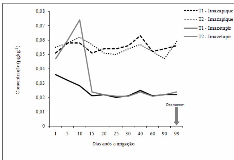
Figura 3. Dissipação de imazaquique e de imazetapir na água de irrigação e de drenagem (99 DPI) do T 1 e T 2 . Embrapa Clima Temperado, Pelotas, RS. 2009.
