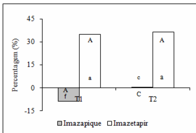
Figura 2. Diferença percentual do residual ( \mu\text{g kg}^{-1} ) entre T 1 e T 2 para o imazaquique (A,C) e imazetapir (A,A), entre imazaquique e imazetapir no T 1 (f, a) e entre imazaquique e imazetapir no T 2 (a, c). Médias seguidas com letras distintas diferem significativamente pelo teste de Duncan 5%. Embrapa Clima Temperado, Pelotas, RS. 2009.
